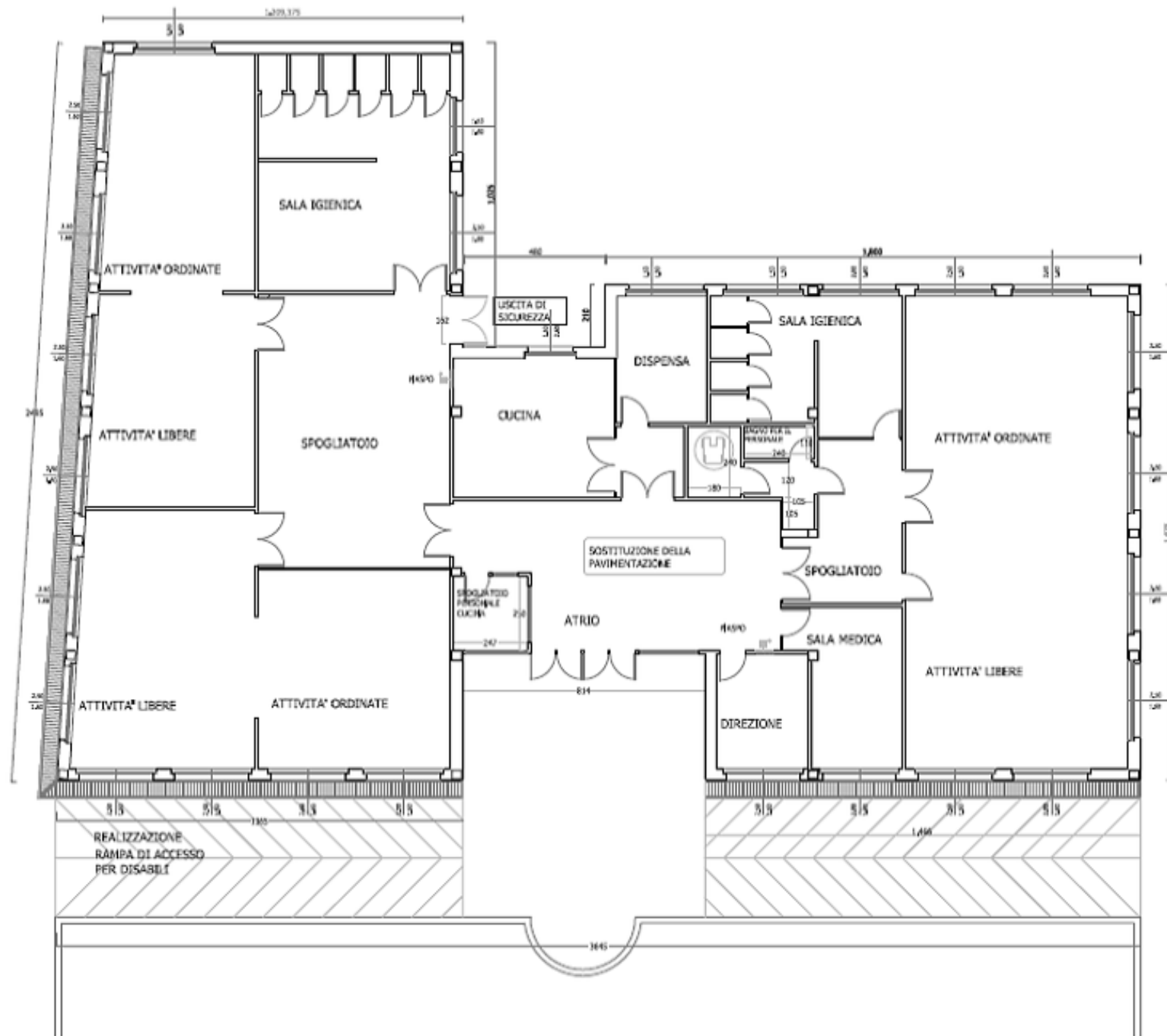
PIANTA PIANO RIALZATO
