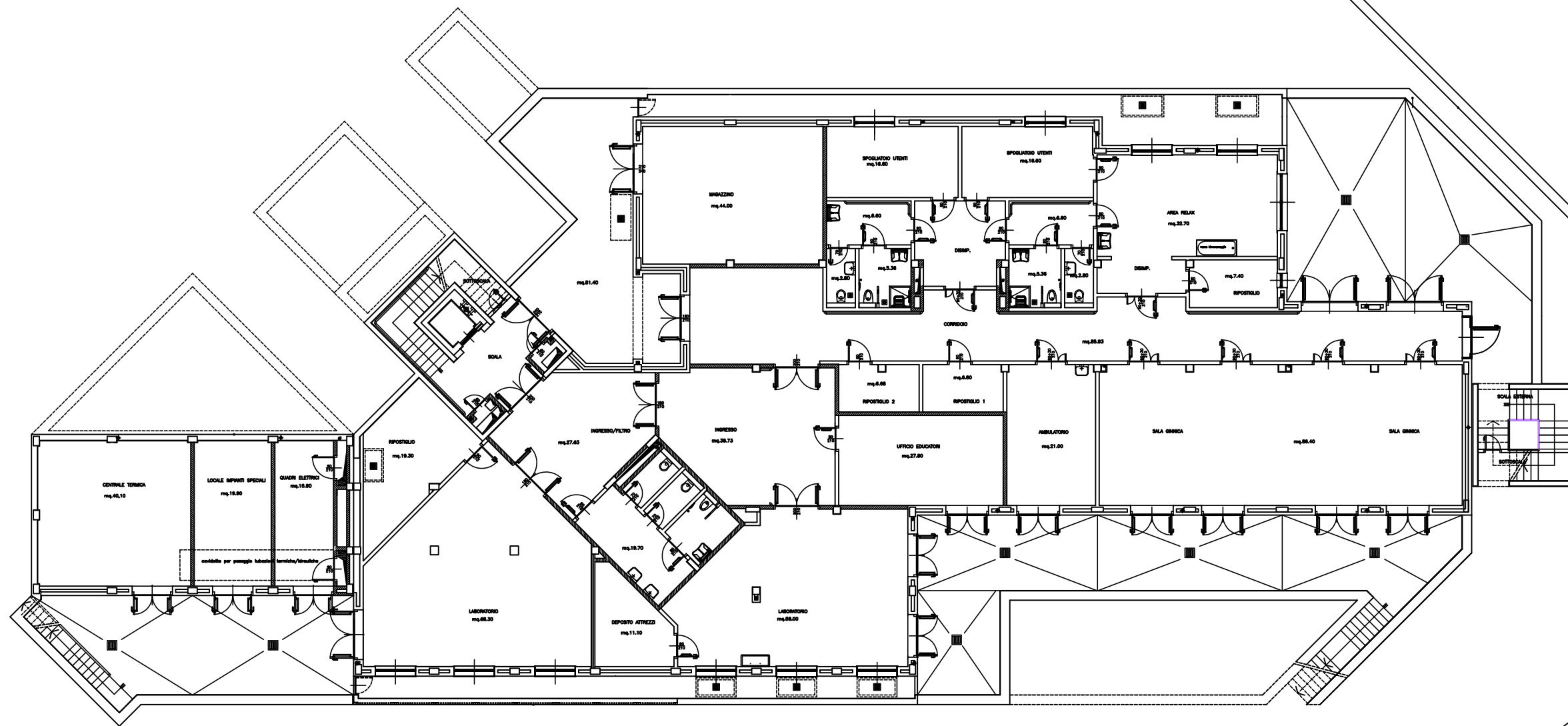
PIANTA PIANO SEMINTERRATO
