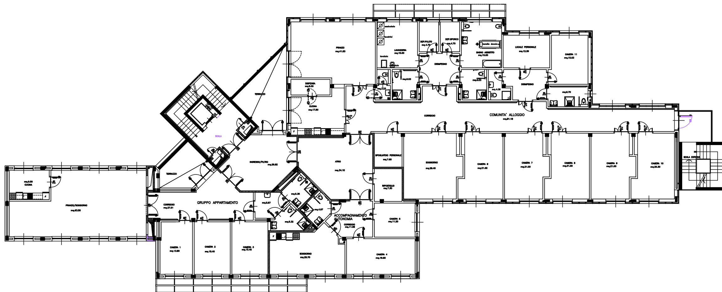
PIANTA PIANO PRIMO (2° PIANO FUORI TERRA)
