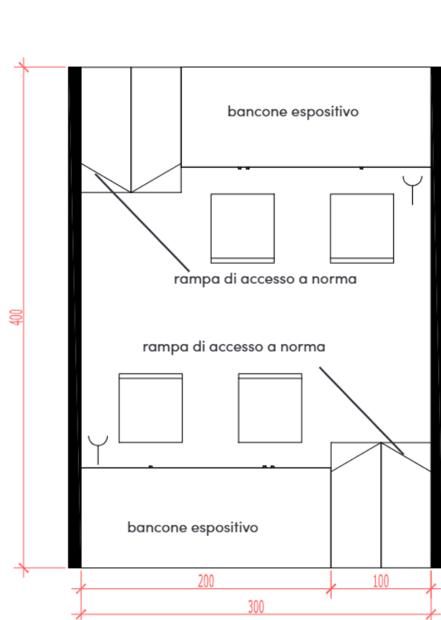
Pianta
